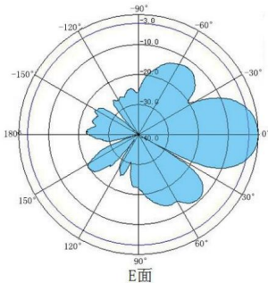
信号方向图
